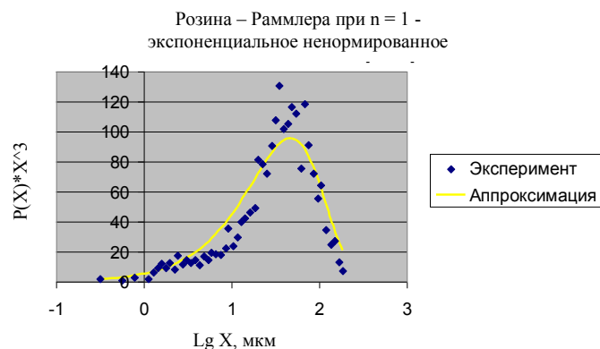
Рис. 6. Аппроксимация экспериментальных данных экспоненциальным распределением
