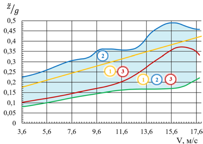
Рис. 3. Результаты инженерной оценки динамики комбайна
