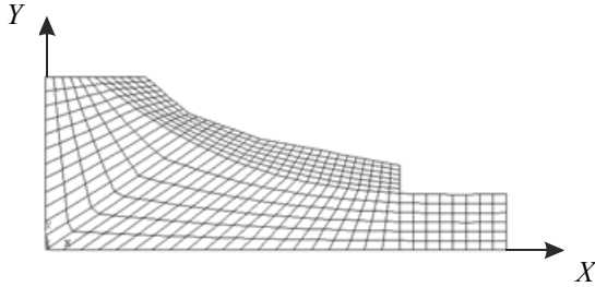
Рис. 3. Конечно-элементная модель склона
