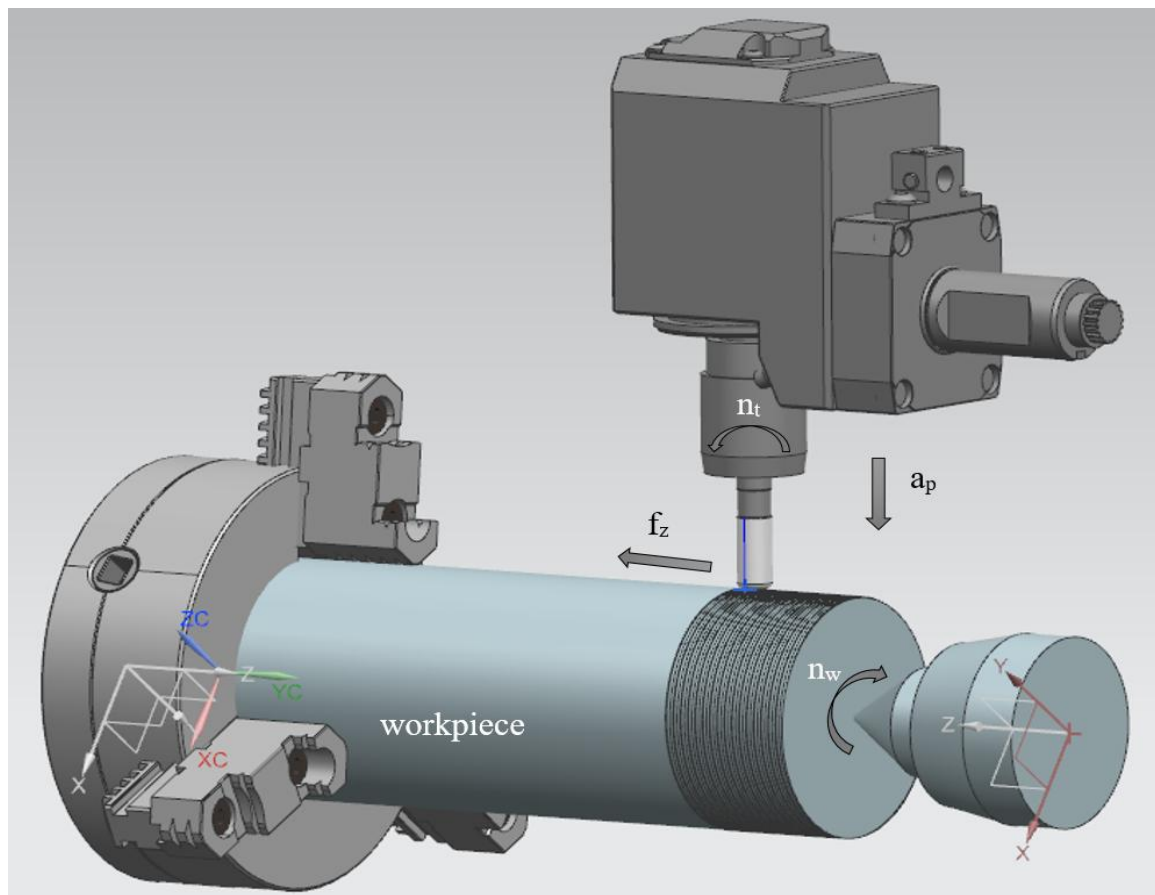
Рис. 2. Схема ортогональной обработки монолитной фрезой YG-1 GMG19910
