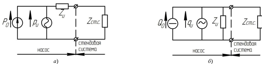
Рис. 1. Модели насоса в виде эквивалентного источника колебаний: а — давления; б — расхода с присоединенной системой: Q_0, P_0 — средний расход и давление; P_u, Q_u — собственная пульсационная производительность насоса по давлению и расходу, Z_u, Z_{cm.c.} — импеданс насоса и стендовой системы (адаптировано из [4])
