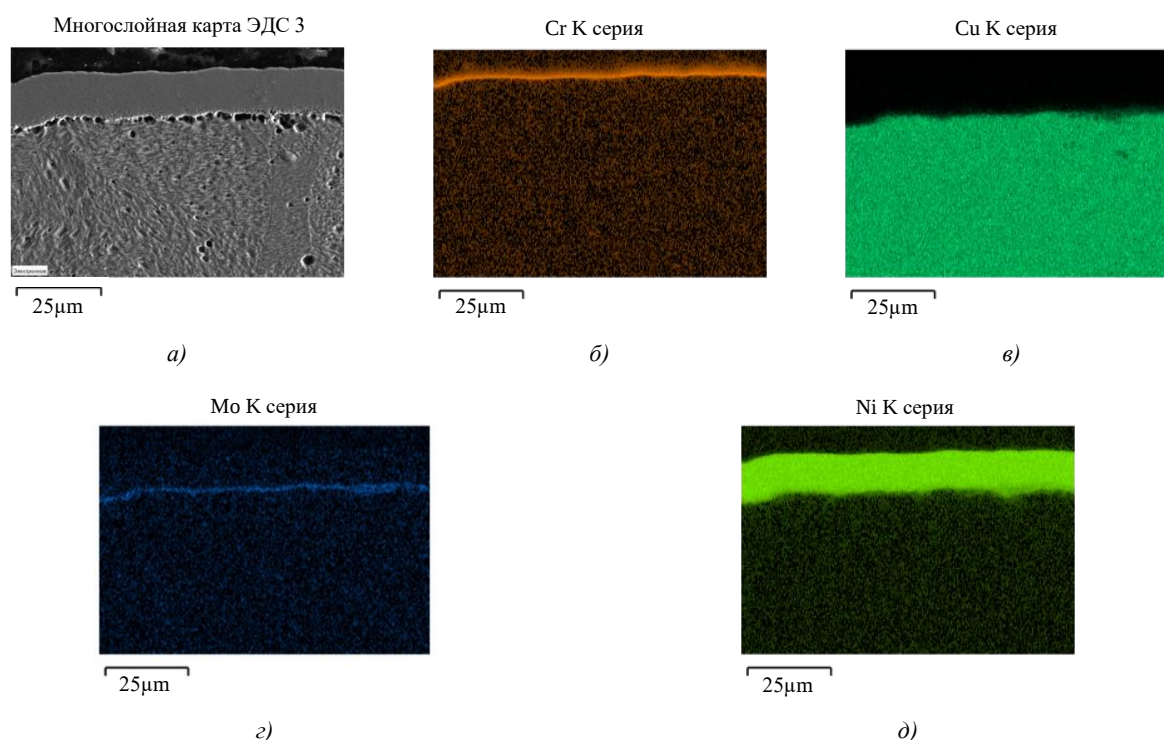
Рис. 5. Цветовые карты распределения химических элементов по глубине покрытия Mo-Ni-Cr, EDAX: а — общий вид покрытия в поперечном сечении (SEM); б–д — распределение элементов на снимке общего вида Cr (б), Cu (в), Mo (г), Ni (д)
