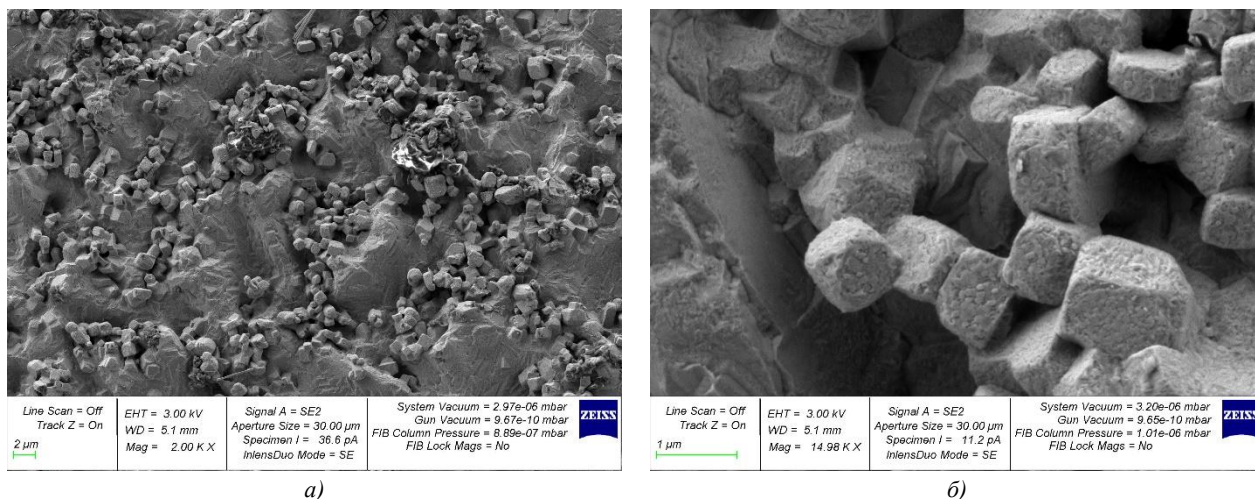
Рис. 8. Медная поверхность образца, оксидированного при температуре 650 °С, SEM: а — расположение кристаллов CuO на поверхности меди; б — морфология кристаллитов CuO
