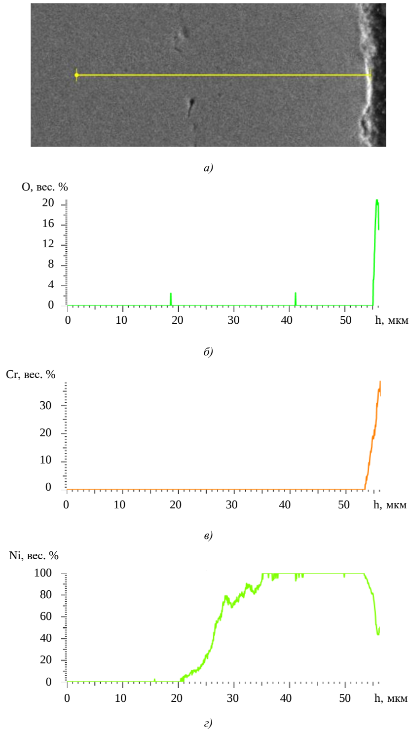
Рис. 11. Распределение основных химических элементов в покрытии Mo-Ni-Cr по глубине h после нагрева до 850 °С, EDAX: а — покрытие в сечении, показано направление сканирования (SEM); б–г — содержание элементов по направлению сканирования: б — кислорода; в — хрома; г — никеля
