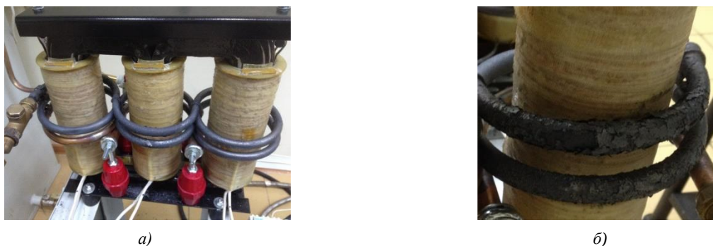
Рис. 1. Экспериментальный индукционный пароперегреватель с медным паропроводом: а — общий вид; б — наиболее сильно окисленные участки паропровода (змеевика) на выходе пара
