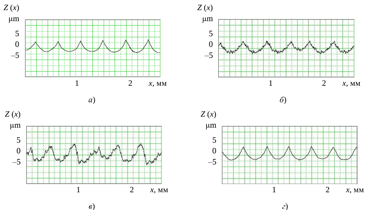
Рис. 2. Профилограммы поверхностей, полученные при различных траекториях формообразования при \Gamma = 35^\circ - 45^\circ : a — попутное фрезерование; b — встречное фрезерование; v — фрезерование сверху вниз; z — фрезерование снизу вверх
