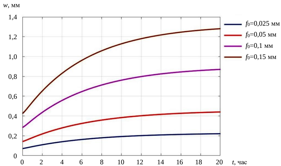
Рис. 5. Кривые изменения прогиба в центре пластины во времени при p = 0,9 p_\infty
