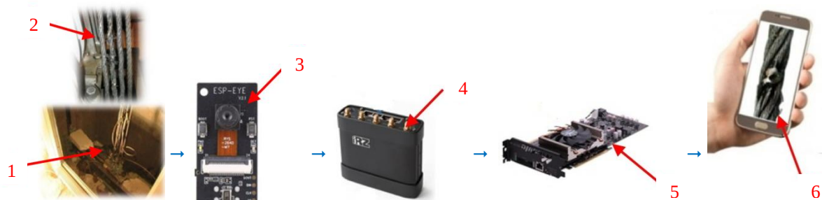
Рис. 2. Функциональная схема ПАК ВИК распознавания дефектов стальных канатов и уравнивающих устройств на основе технологий компьютерного зрения и искусственного интеллекта: 1 — уравнивающее устройство; 2 — дефекты каната; 3 — IP-камера; 4 — GSM-модем; 5 — нейровычислитель; 6 — изображение в мобильном устройстве (рисунок авторов)
