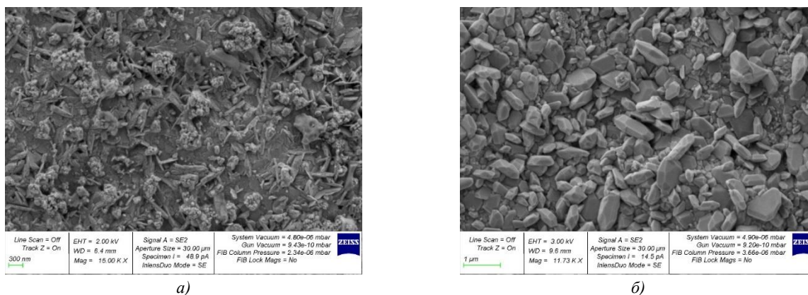
Рис. 9. Поверхность образцов с покрытием \text{Mo-Ni-Cr} , SEM: а — после нагрева до температуры 650 °С; б — после нагрева до температуры 850 °С
