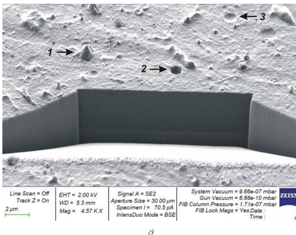
Рис. 2. Субструктурные дефекты ионно-плазменных покрытий системы Ti-Al-N, SEM: а — на поверхности покрытия в нормальной проекции (показаны стрелками); б–г — на поверхности покрытия и в сечении кросс-секции FIB
