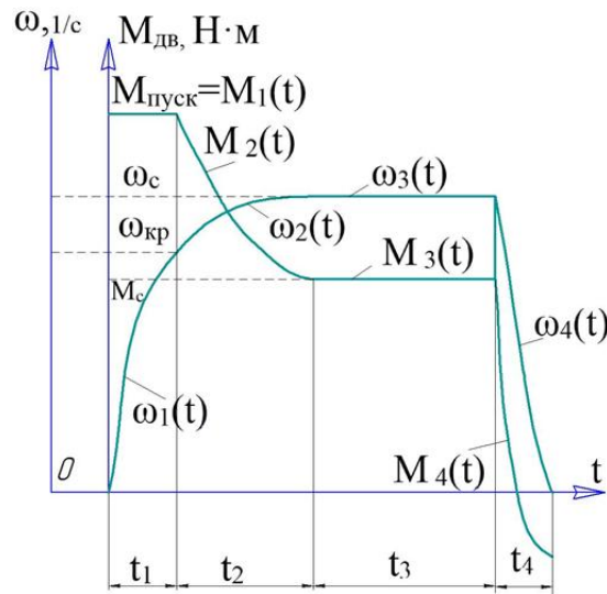
Рис. 6. Качественная картина изменения угловой скорости \omega(t) и момента на валу двигателя M_{дв}(t) по периодам движения лифта
